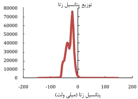
شکل 2 توزیع پتانسیل زتا برای نمونه 1:1 صمغ عربی - نانولوله کربنی
