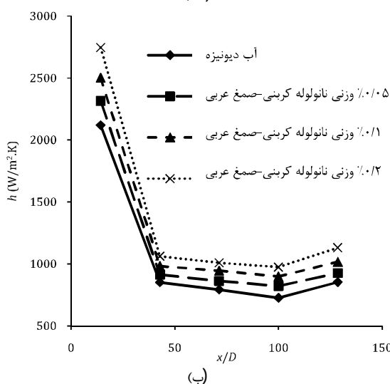
شکل 6 ضریب انتقال حرارت جابجایی محلی بر اساس طول بدون بعد لوله، الف) Re=2000\pm 50 و ب) Re=800\pm 50
