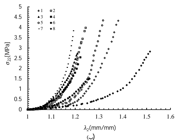
شکل 2 نمودار تنش-کشش برای نمونه‌های صافن انسان. الف) تنش و کشش در راستای پیرامونی (11) و ب) تنش و کشش در راستای طولی (22)
