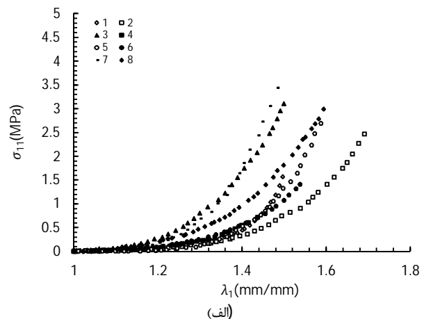
شکل 3 نمودار تنش-کشش حاصل از ضرایب مونی - ربولین الف) در راستای پیرامونی و ب) راستای طولی ( \lambda_1 = \lambda_2 = \lambda )
