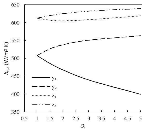
شکل 15 تغييرات ضريب انتقال حرارت جابجايي میانگين با Q_r بر روی دیواره‌های مختلف کانال برای حالت AR = 0.5 و \phi = 1.5\% ، Gr = 5 \times 10^5 ، Re = 700
