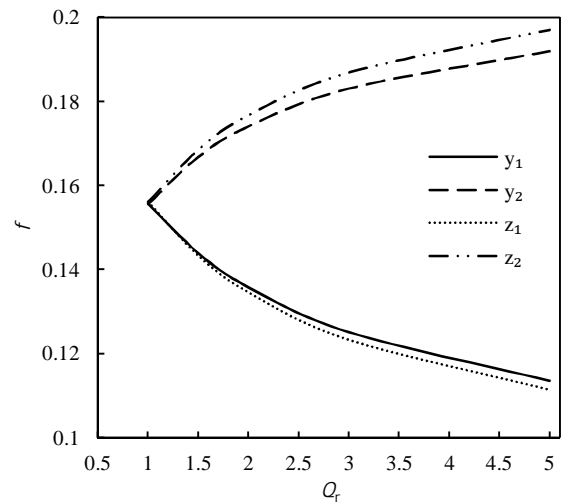
شکل 14 تغييرات ضريب اصطکاک میانگين با Q_r بر روی دیواره‌های مختلف کانال برای حالت AR = 0.5 و \phi = 1.5\% ، Gr = 5 \times 10^5 ، Re = 700
