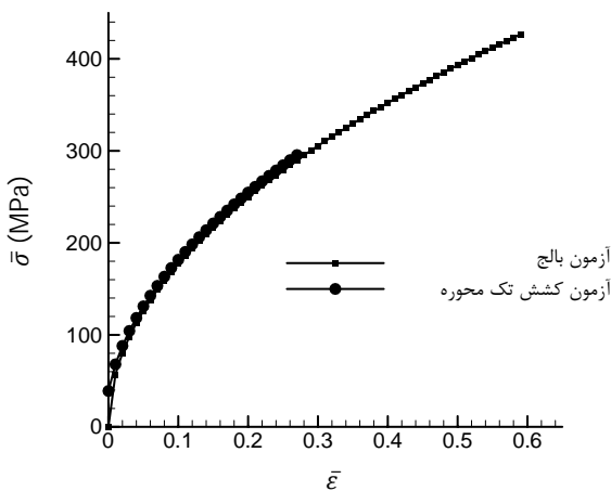
شکل 11 نتایج آزمون بالج و آزمون کشش با در نظر گرفتن ناهمسانگردی
