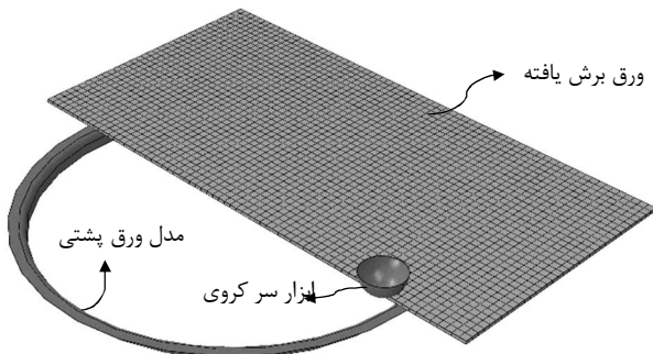
شکل 6 برشی از مدل تعریف‌شده در نرم‌افزار آباکوس
