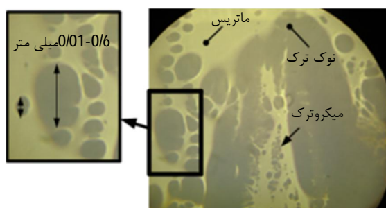
شکل 13 میکروساختار کامپوزیت کربن-اپوکسی تک جهت
