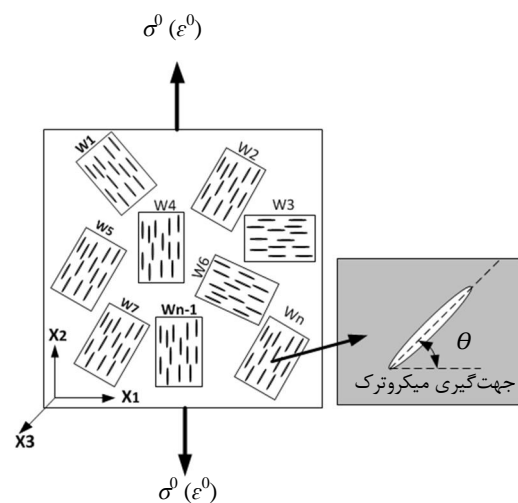
شکل 6 جهت گیری دسته‌های میکروتُرک در المان حجمی معرف
