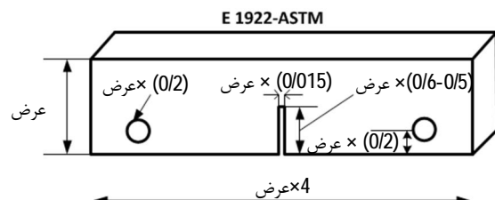
شکل 14 نمونه استاندارد شکست ASTM-E1922
