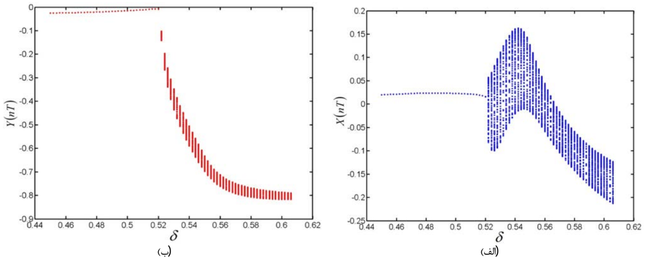
دیگرام دوشاخه‌گی، یاتاقان دولب، \lambda = 1.5 ، \bar{p} = 0.001
