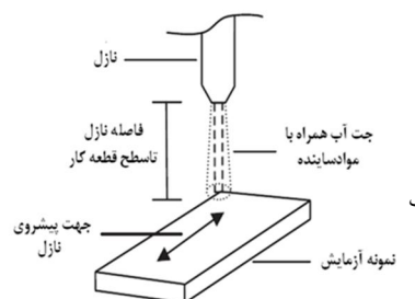
شکل 4 (الف) آماده سازی آزمایش (ب) نمایش شماتیک متغیرهای آزمایش
