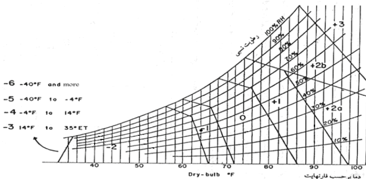
شکل ۲: محدوده ضرایب راحتی، بر حسب شاخص ترچونگ
