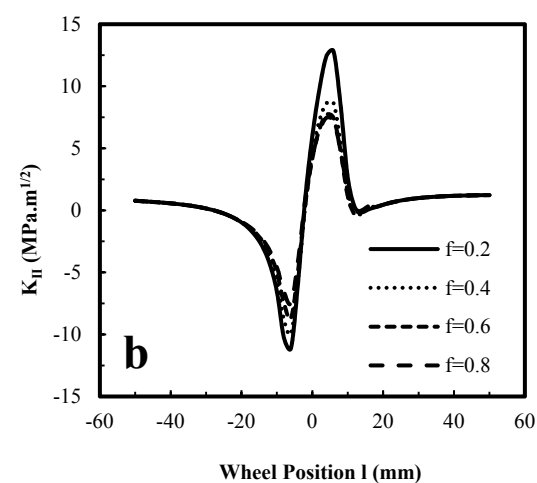
شکل ۱۶- روند تغییرات ضریب شدت تنش به ازای ضرایب اصطکاک مختلف K_I (a) و K_{II} (b)
