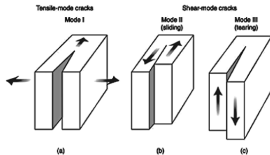
شکل ۱- انواع مد بارگذاری ترک
