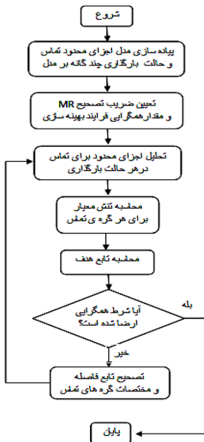
شکل ۳- فلوجارت بهینه سازی شکل تماس
