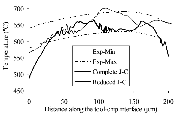
شکل ۹- تغییرات دما در امتداد ناحیه برش ثانویه
