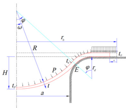
شکل ۲- فرآیند هیدروفرمینگ ورق در حالت نیروی ورق گیر کم، ورق در حالت اولیه (خط چین) و ورق تغییر شکل یافته (خط پر)
