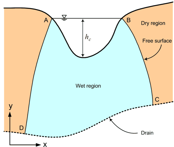
شکل ۱- طرح شماتیکی از مقطع یک کانال روباز و نشت سیال در بستر کانال و تشکیل نواحی تر و خشک و سطح آزاد آب
