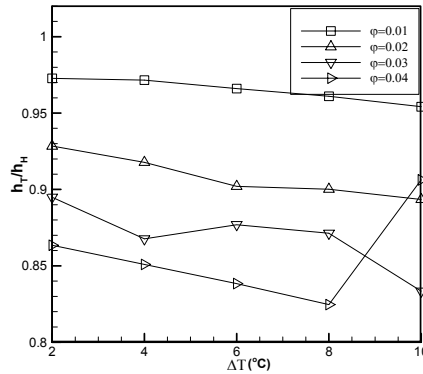
شکل ۴- تغییرات نسبت ضریب جابه‌جایی متوسط دو مدل انتقال و همگن برحسب اختلاف دما برای کسر حجمی‌های مختلف
