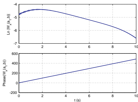
شکل (۳): نمودار اندازه و فاز تبدیل ویولت پاسخ به ازا a_1=180
