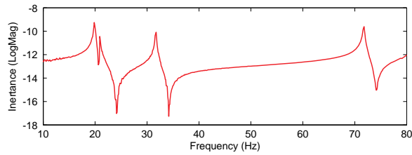
شکل (۵): نمودار پاسخ فرکانسی سازه
