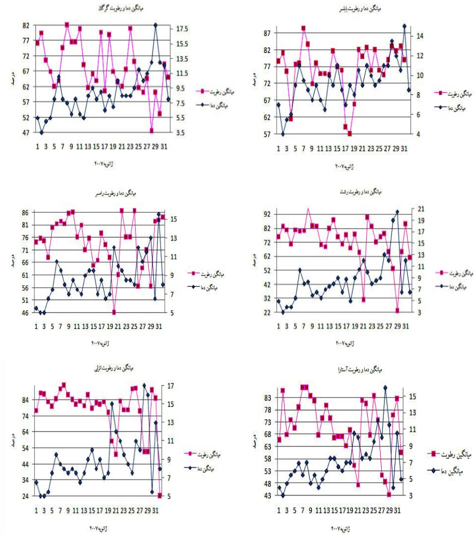
شکل ۳ مقایسه دما و رطوبت روزانه ایستگاه‌های سواحل خزر؛ زمایه ۲۰۰۷
