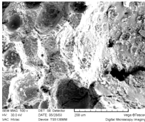
(ب): Cu-28Zn، ۸/۲ میلی متر از بالا
