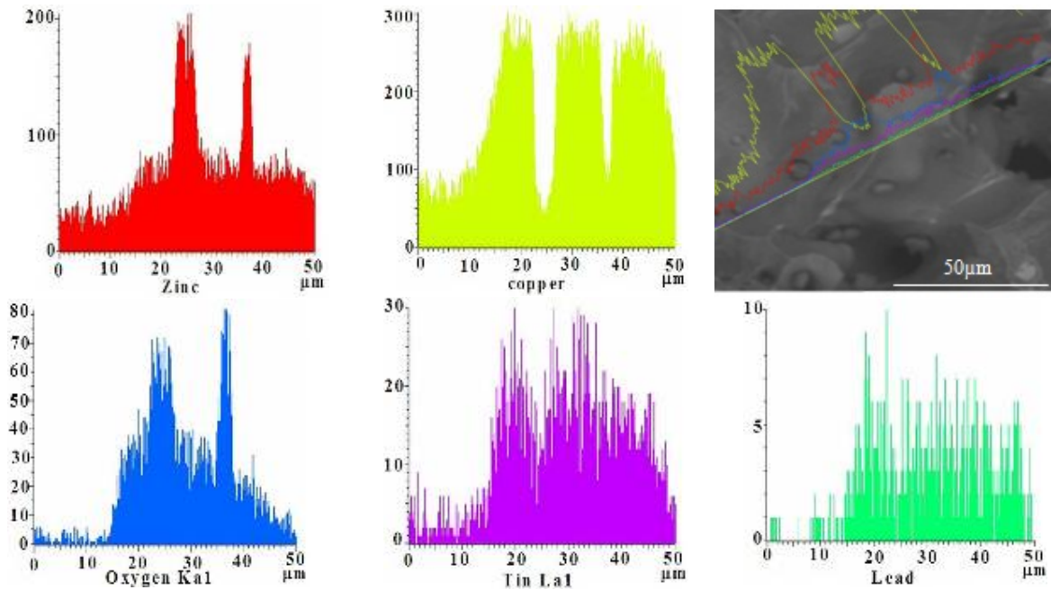
شکل ۱۰- نتایج آنالیز خطی مناطق مرزدانه‌ای سطح شکست نمونه Cu-20Zn
