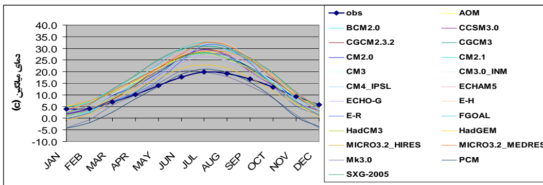
شکل ۷- مقایسه‌ی کیفی نتایج شبیه‌سازی داده‌های میانگین شبیه‌های GCM با داده‌های مشاهده‌ای.
