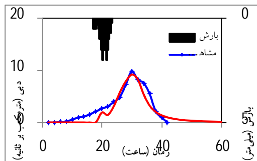
شکل 5- آبنمای مشاهداتی و شبیه‌سازی شده‌ی رویداد
