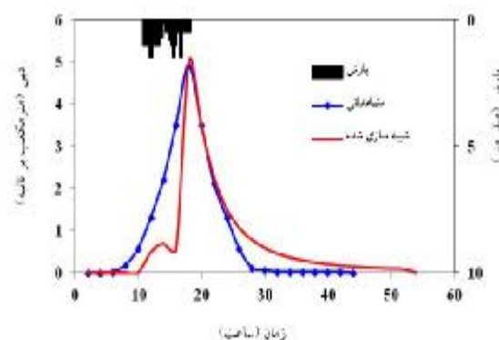
شکل 9- اعتبارسنجی شبیه‌سازی با رویداد مورخ 23 و 24/8/1372
