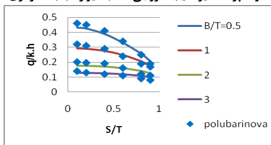
شکل ۱۴- مقایسه بدهی نشت از زیر سد ناتراوا با سپر ورقه ای قرینه واقع بر پی همگن با ژرفای متناسبی با نتایج پولوبارینووا- کوچینا.
