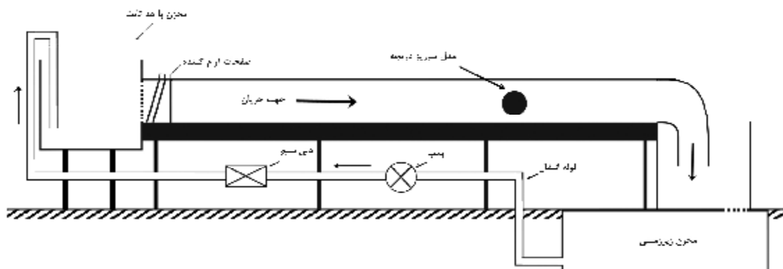
شکل (1) اجزای نهر پایه‌دار آزمایشگاهی مورد استفاده.
