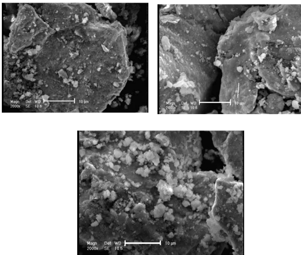
شکل ۲- تصاویر میکروسکوپی الکترونی روبشی از پودر کامپوزیتی آلیاژ پایه کبالت حاوی: (الف) ۱۰ درصد وزنی فورستريت، (ب) ۱۵ درصد وزنی فورستريت، (ج) ۲۰ درصد وزنی فورستريت
