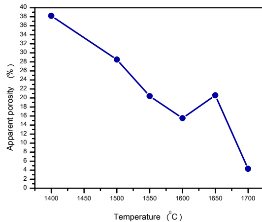
شکل ۶- تغییرات تخلخل ظاهری نمونه در دماهای مختلف زینتر
