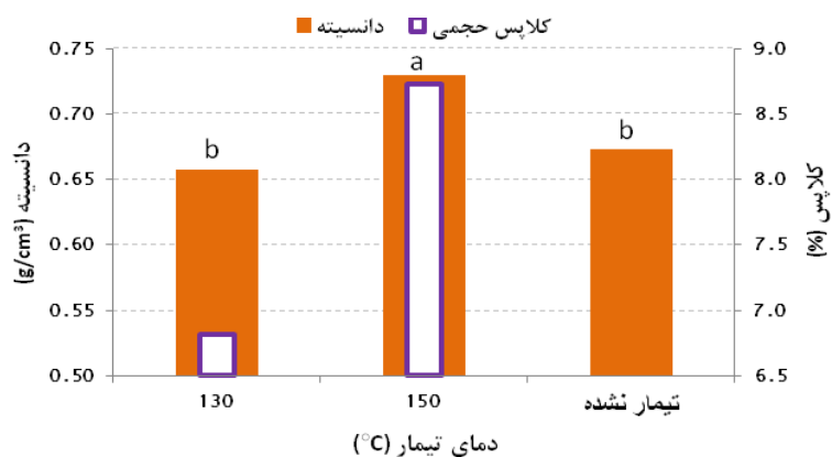
شکل ۲- اثر دمای تیمار گرمایی بر چگالی و چین خوردگی حجمی چوب راش؛ حرف‌های a و b نشان دهنده گروه بندی دانکن به ترتیب بزرگ‌ترین و کوچک‌ترین مقادیر چگالی می‌باشند.
