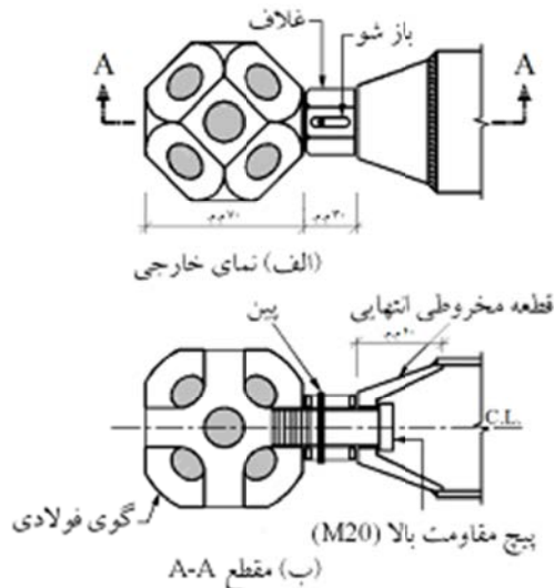
شکل ۲- جزئیات سیستم اتصال گویسان
