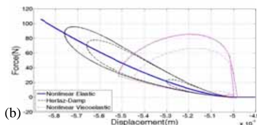
شکل ۳- (a) منحنی نیرو- تغییر شکل المان‌های خطی و (b) منحنی نیرو- تغییر شکل المان‌های غیر خطی
