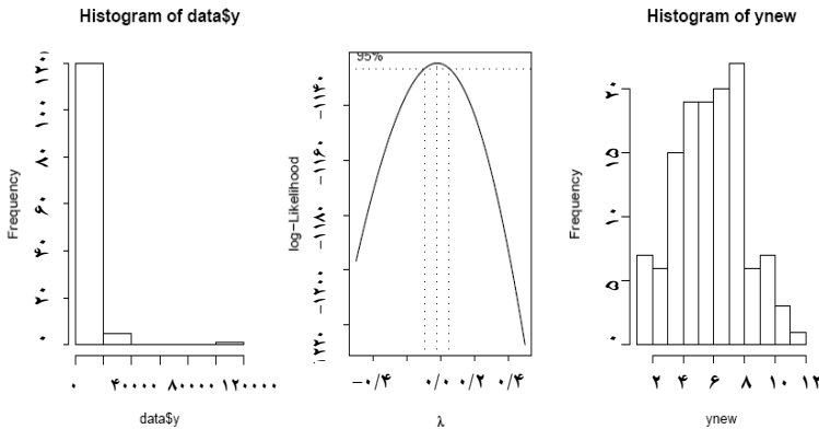
شکل ۲ فرض نرمالیتی
