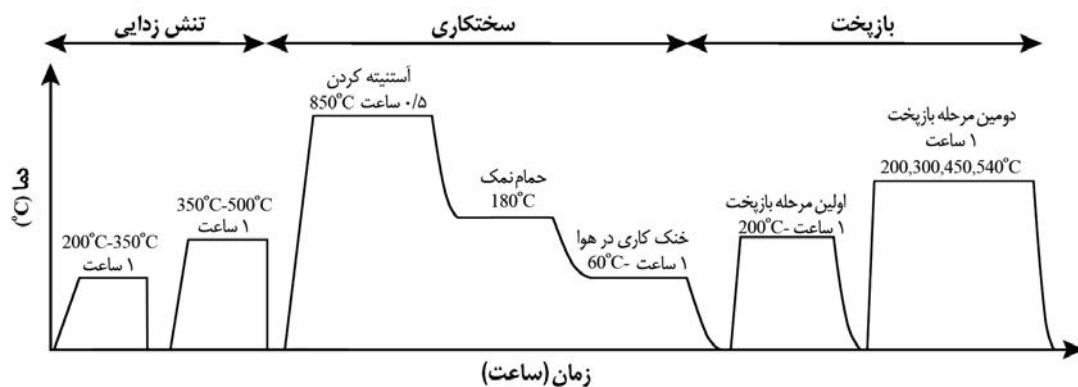
شکل (۱) فرایند عملیات حرارتی فولاد AISI ۴۱۴۰.
