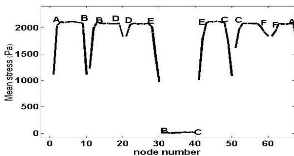
شکل (۹): توزیع تنش متوسط در جداره مقطع مستطیلی با دو سلول
