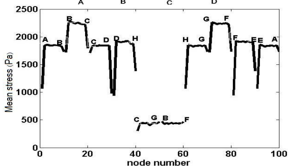
شکل (۱۰): توزیع تنش متوسط در جداره مقطع مستطیلی با سه سلول
