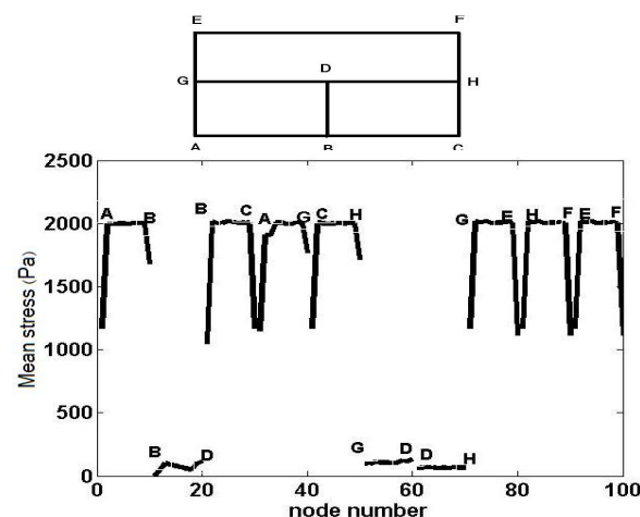
شکل (۱۲): توزیع تنش متوسط در جداره مقطع مستطیلی با سه
