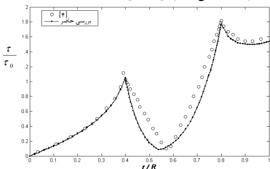
شکل (۱۳): مقایسه نتایج حاصل برای مقطع چهار سلولی دایره ای
