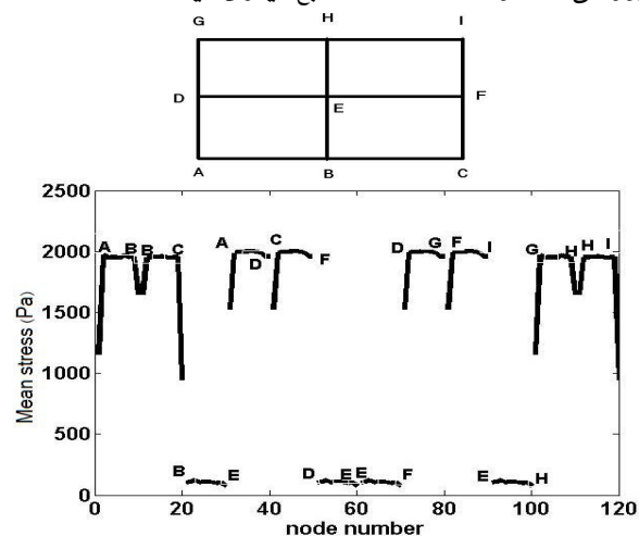
شکل (۱۱): توزیع تنش متوسط در جداره مقطع مستطیلی با چهار
