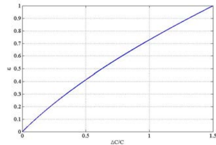
شکل (۴): منحنی تغییرات \mathcal{E} در برابر پارامتر \frac{\Delta C}{C} .
