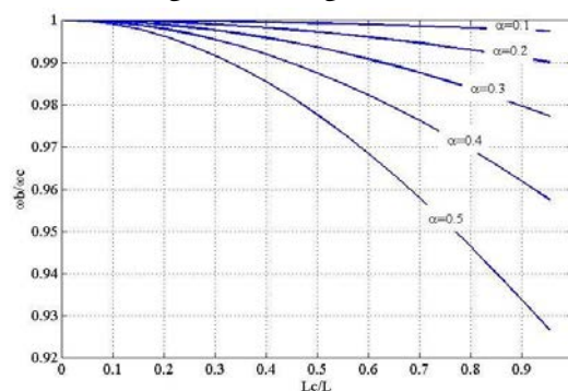
شکل (۹): تغییرات نسبت فرکانسی تیر یکسرگیردار ترک‌دار در برابر تغییر موقعیت نسبی ترک به ازای مقادیر مختلف شدت ترک.
