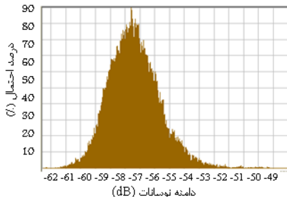
شکل (۶): منحنی هیستوگرام در شرایط پایدار
