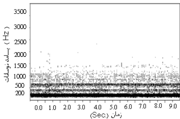
شکل (۹): نمودار اسپکتروال در شرایط ناپایدار
