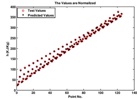
شکل (۱۲): ارزیابی شبکه عصبی آموزش داده شده با داده‌های نرمالیزه برای آنتالپی
