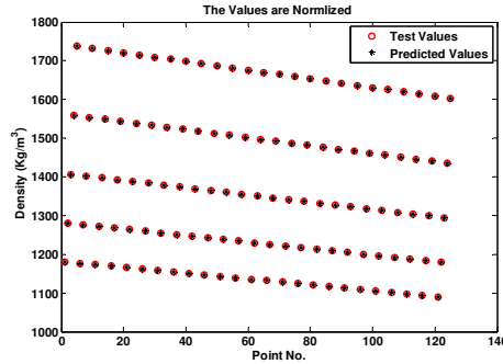
شکل (۱۰): ارزیابی شبکه عصبی آموزش داده شده با داده‌های نرمالیزه برای چگالی
