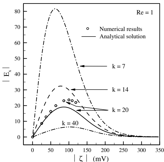
شکل ۷. تغییرات قدرت میدان الکتریکی القایی در برابر قدرمطلق زتا پتانسیل، وقتی Re = 1 و k برابر ۷، ۱۴ و ۲۰ و ۴۰ است.
