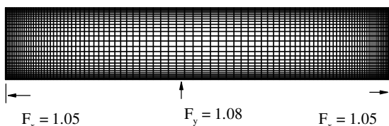
شکل ۲. یک شبکه معمولی بکار رفته در ریزمجرای تخت.
