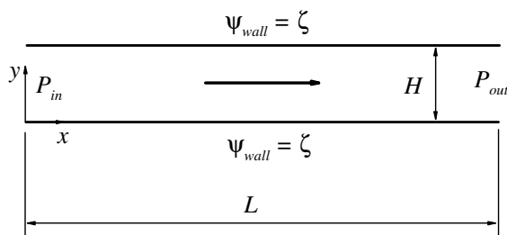
شکل ۱. طرحواره هندسه جریان فشار- محرک در ریزمجرای تخت صفحه موازی
