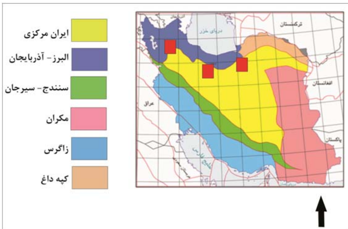
تصویر ۱- موقعیت قرارگیری مهم‌ترین زون‌های زئولیتی ایران، علامت ستاره (نبوی ۱۳۵۵)
