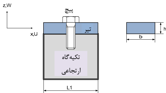
شکل ۲ قسمت مستقر بر روی تکیه‌گاه اصطکاکی تیر
