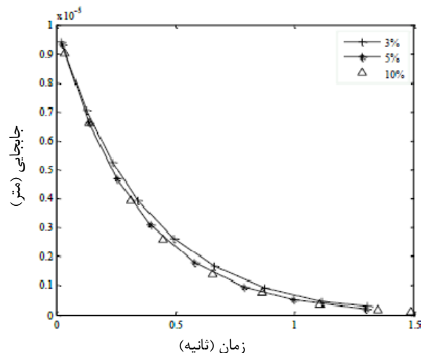
شکل ۱ پاسخ زمانی ارتعاشات آزاد تیر یک سر آزاد با ذرات نانو
