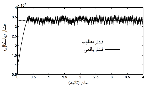
شکل ۵ تعقیب فشار مرجع در حالتی که از تابع \text{sgn}(s) در الگوریتم کنترلی مد لغزشی استفاده شده است
