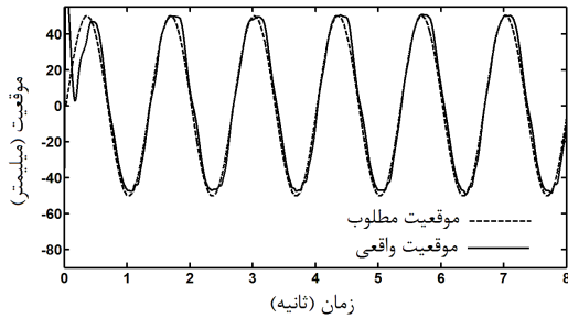
شکل ۲۲ تعقیب مسیر سینوسی با فرکانس ۰/۷۵ هرتز در سیستم تحت کنترل امپدانس در فضای آزاد با سفتی هدف ۴۰۰۰ نیوتن بر متر، میرایی هدف ۳۰ نیوتن ثانیه بر متر و اینرسی هدف ۴/۵ کیلوگرم
