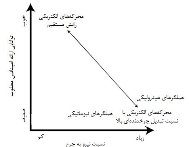
شکل ۱ مقایسه انواع عملگرها از لحاظ توانایی ارائه امپدانس مورد نظر
