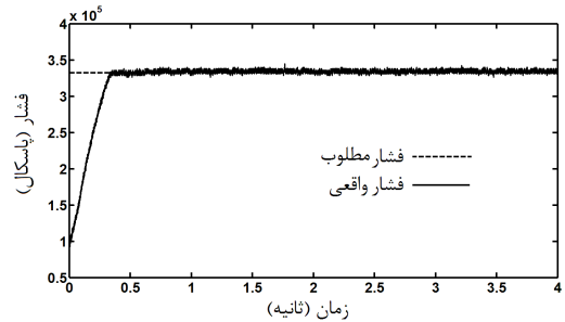
شکل ۶ تعقیب فشار مرجع در حالتی که از تابع \text{sat}(s/\theta) در الگوریتم کنترلی مد لغزشی استفاده شده است
