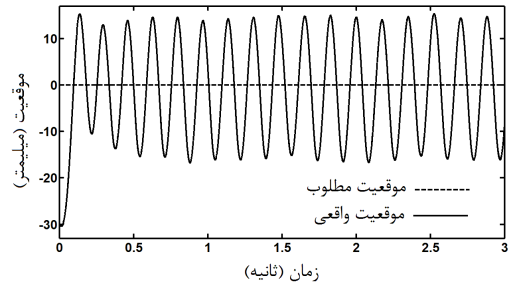
شکل ۱۷ تعقیب موقعیت در سیستم تحت کنترل امپدانس در فضای آزاد با سفتی هدف ۴۰۰۰ نیوتن بر متر، میرایی هدف ۳۰ نیوتن ثانیه بر متر و اینرسی هدف ۱/۸ کیلوگرم
