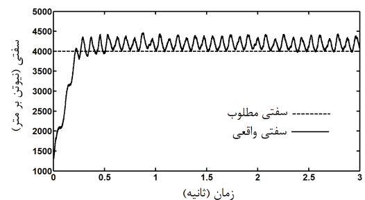
شکل ۲۰ تعقیب سفتی در سیستم تحت کنترل امپدانس با سفتی هدف ۴۰۰۰ نیوتن بر متر، میرایی هدف ۳۰ نیوتن ثانیه بر متر و اینرسی هدف ۱/۸ کیلوگرم
