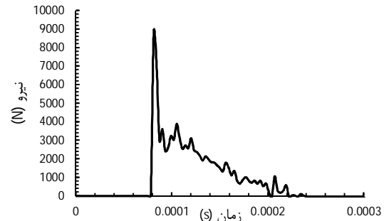
شکل 20 تغییرات نیروی پرتابه
