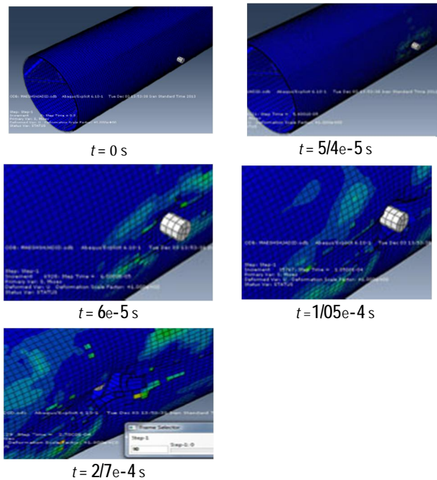
شکل 12 بررسی زمانی نفوذ پرتابه
