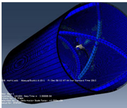
شکل 17 شبکه تقویت‌کننده متشکل از تقویت‌کننده‌های محیطی و طولی
