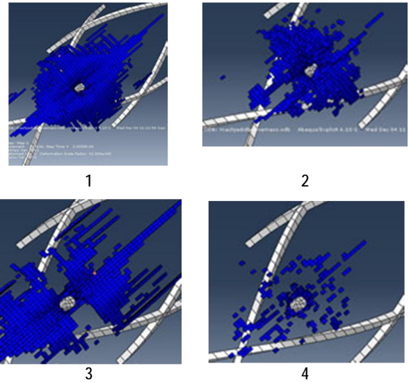
شکل 18 گستردگی سطح آسیب‌دیدگی
