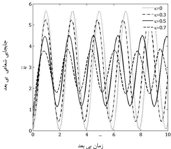
شکل 2 تغییرات زمانی جابجایی شعاعی در نقطه میانی در راستای شعاع
