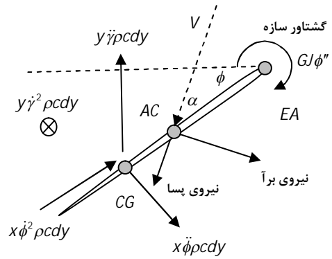
شکل 2 دیاگرام نیروهای وارد به بال در پرنده بال زن
