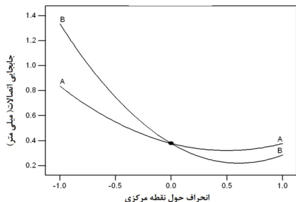
شکل 5 نمودار تغییرات جابه جایی اتصالات برشی تک لبه با تغییر جزئی متغیرهای A و B حول نقطه مرکزی
