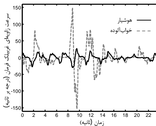
شکل 16 نمودار سرعت زاویه‌ای فرمان برای راننده شماره 5 در دو حالت هوشیار و خواب‌آلوده
