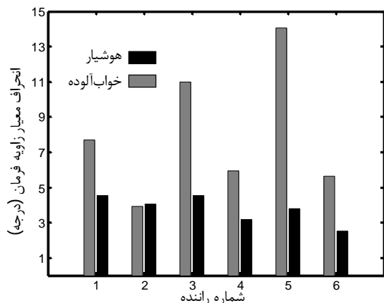
شکل 24 انحراف معیار زاویه فرمان برای همه راننده‌ها (1 تا 6)
