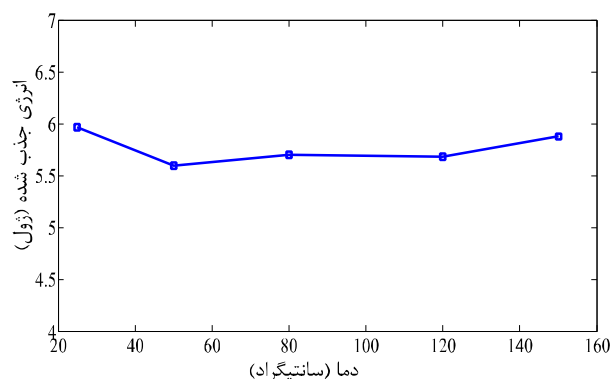
شکل 11 تغییرات انرژی جذب شده در دماهای مختلف و انرژی ضربه 6/87 ژول
