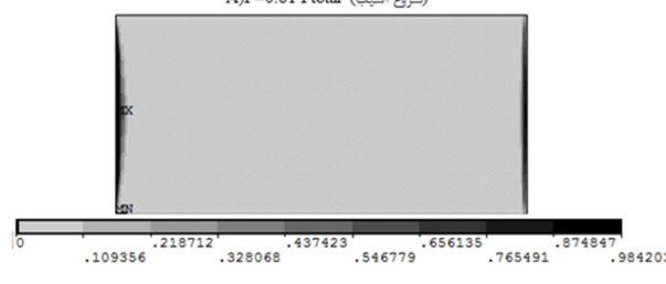
شکل 9 توزیع متغیر آسیب در سطح مشترک پوسته - تقویت کننده نمونه A
