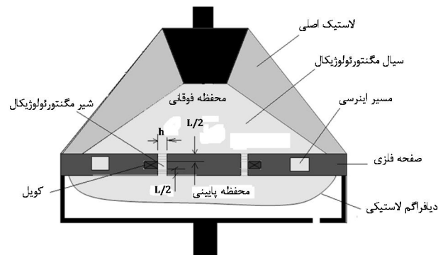
شکل 3 شماتیک دسته موتور مگنتورولوزیکال (طرح برگرفته شده از ایده مرجع [14])
