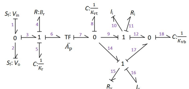
شکل 4 مدل باند گراف دسته موتور مگنتورولوزیکال
