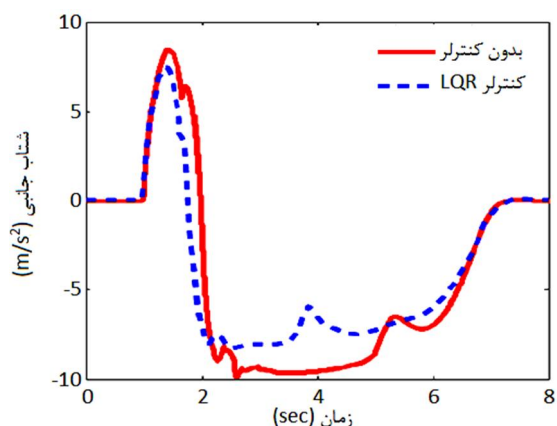
شکل 5 شتاب جانبی در مانور قلاب ماهی (زاویه فرمان 5 درجه)
