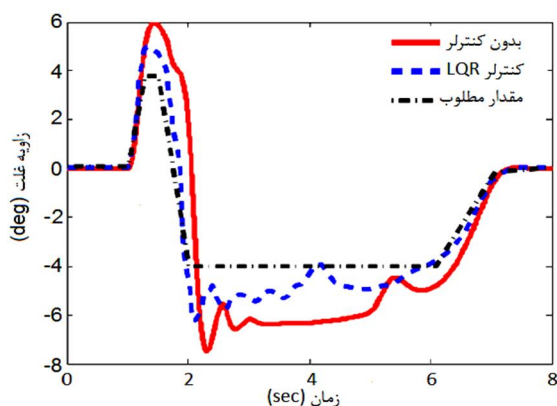
شکل 6 زاویه غلت در مانور قلاب ماهی (زاویه فرمان 5 درجه)
