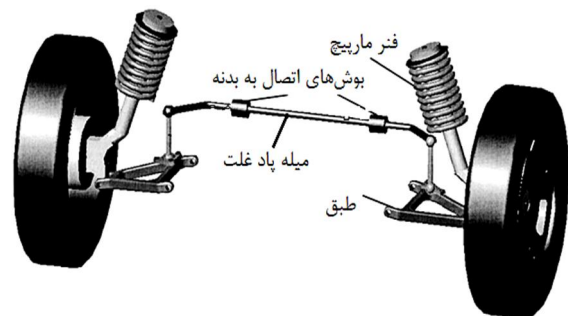
شکل 1 میله پاد غلت و محل اتصال آن
