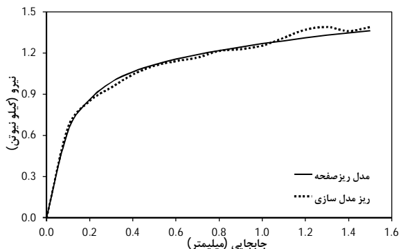
شکل 10 نمودار نیرو-جابجایی نمونه تحت بارگذاری دومحوری
