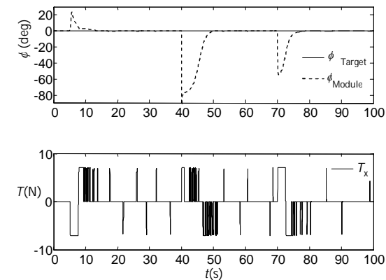
شکل 13 تعقیب فرمان هدایت و فرمان کنترل کانال چرخ با ناهمراستایی تراستر و نویز اندازه‌گیری
