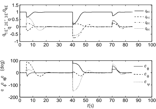
شکل 21 همگرایی بردار کوتاه‌ترین خطا و زوایای اوپلر با ناهمراستایی تراستر و نوبز اندازه‌گیری در تست HIL
