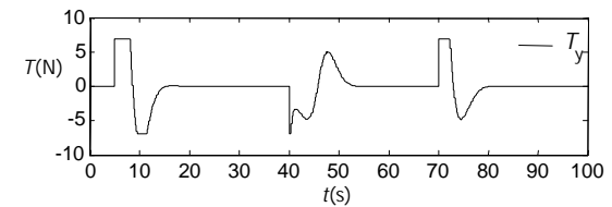
شکل 8 تعقیب فرمان هدایت و فرمان کنترل کانال چرخ
