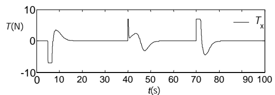
شکل 9 تعقیب فرمان هدایت و فرمان کنترل کانال فرار در زاویه 90 درجه
