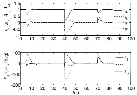
شکل 16 همگرایی بردار کوتاه‌ترین خطا و زوایای اوپلر با ناهمراستایی تراستر و نوبز اندازه‌گیری
