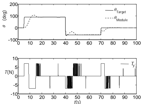
شکل 14 تعقیب فرمان هدایت و فرمان کنترل کانال فرار با ناهمراستایی تراستر و نویز اندازه‌گیری در زاویه 90 درجه
