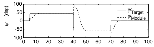
شکل 9 تعقیب فرمان هدایت و فرمان کنترل کانال فرار در زاویه 90 درجه
