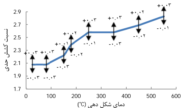
شکل 13 تغییرات نسبت کشش حدى در دماهای مختلف شکل‌دهی
