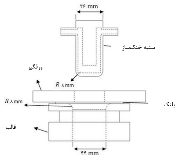
شکل 2 هندسه ابزاربندی
